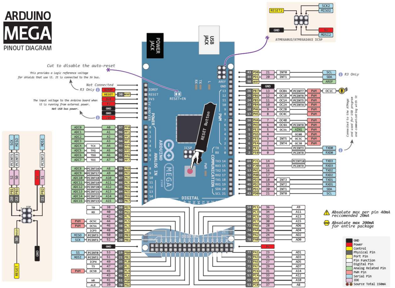
Obrázek 7.3. Arduino Mega
