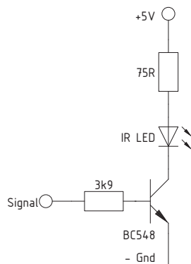
Obrázek 3.1. Příklad na 50mA IR ovladač s ( V_f 1.5V, I_f 100mA,)
