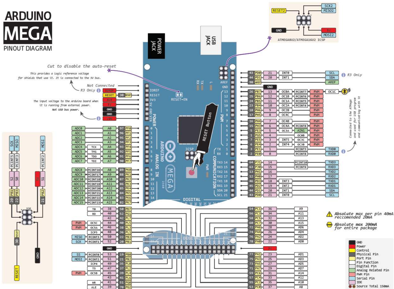
Obrázek 7.3. Arduino Mega
