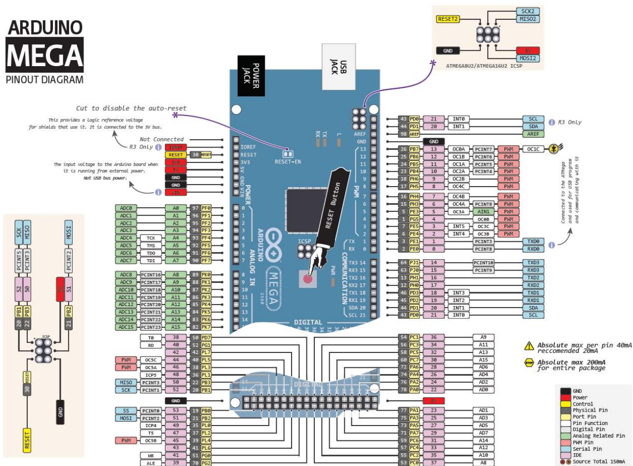
Obrázek 7.3. Arduino Mega
